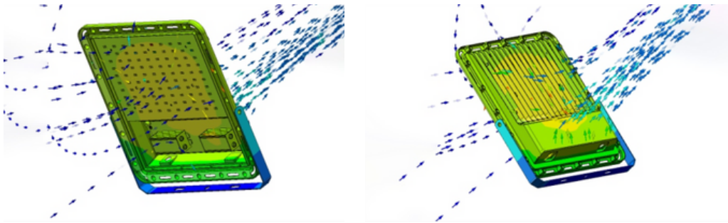
Convección térmica de aire
